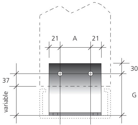
LONG TRIMMER CLEAT
